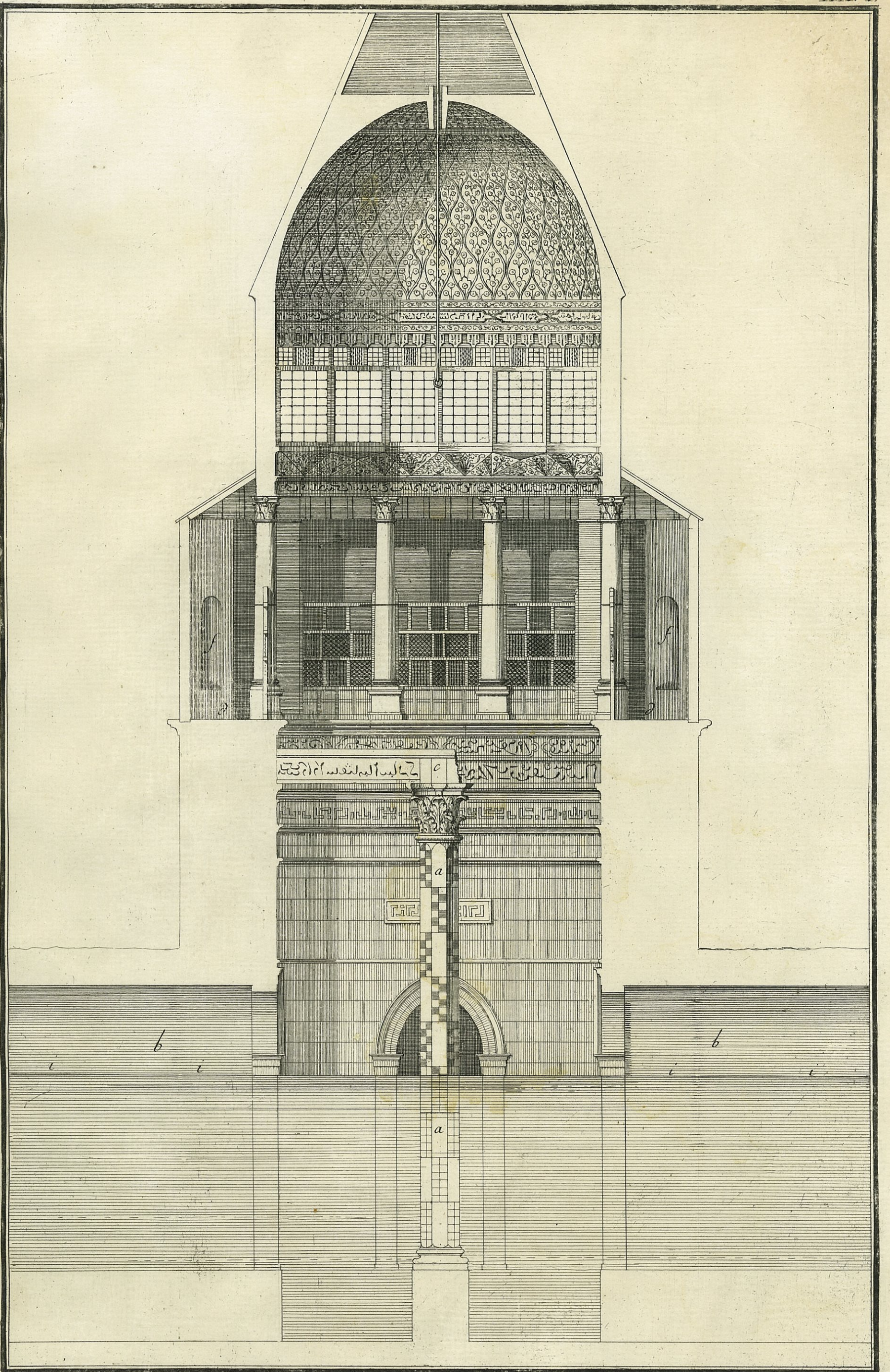
Coupe du Mokkias, à la pointe de l'Isle de Rodda, au Vieux Caire. a, Colonne, dont les différentes mesures marquent combien le Nil hausse et baisse. b, Entrées et Sorties des eaux. c, Architrave sur La dite Colonne. d, Galerie. f, Niches. i Surface du Nil.
